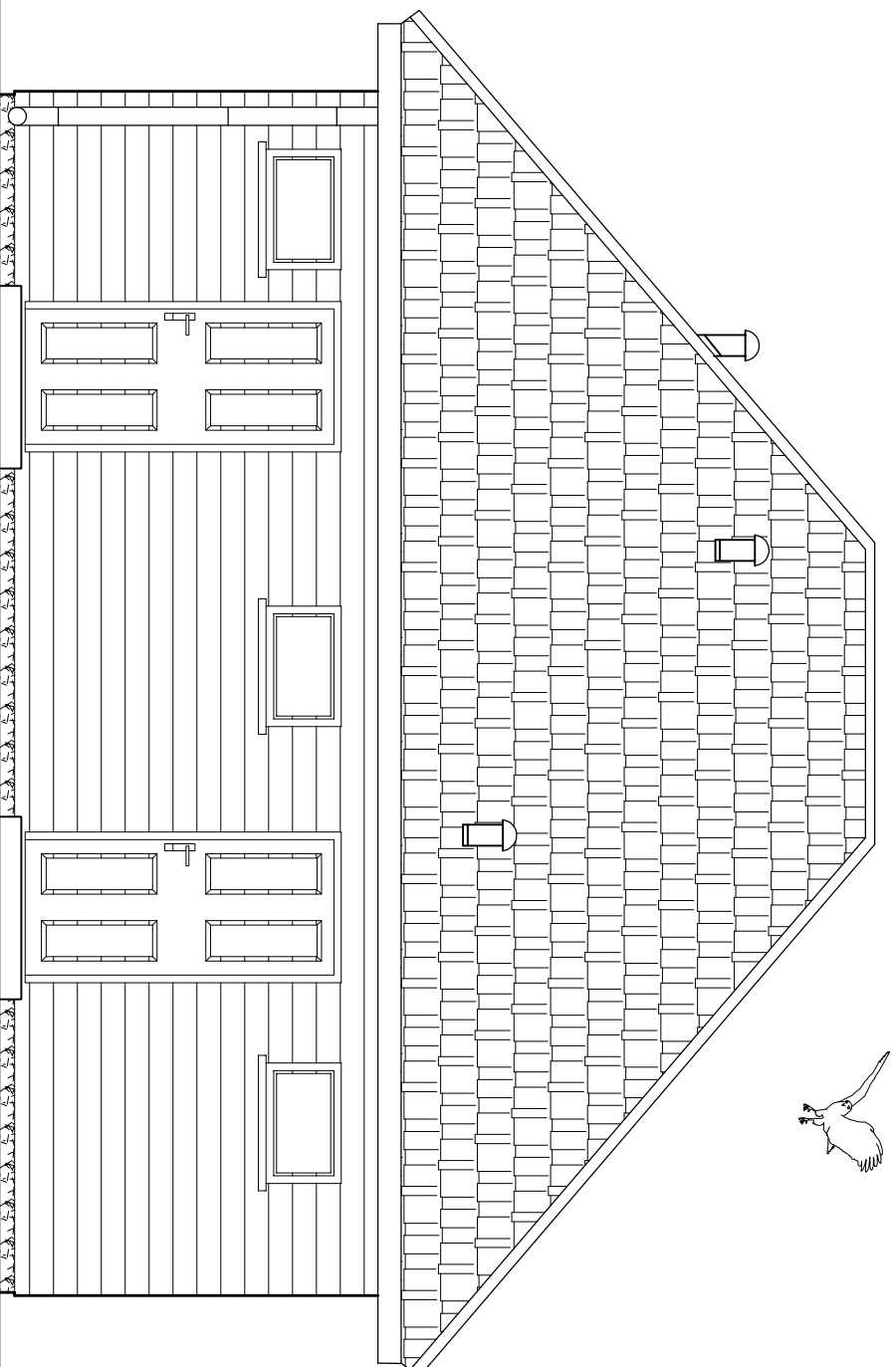
ELEWACJA PÓŁNOCNO - WSCHODNIA
